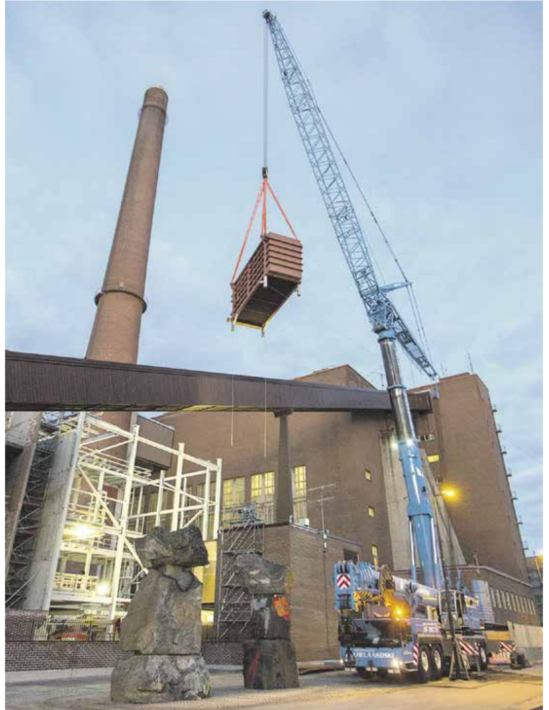
Salmisaareen valmistuvan lämpölaitoksen pellettikattilan osien nostoa.
